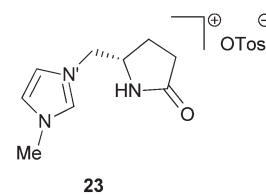
Fig. 5 Chiral bidentate uNHC precursor 23 .
