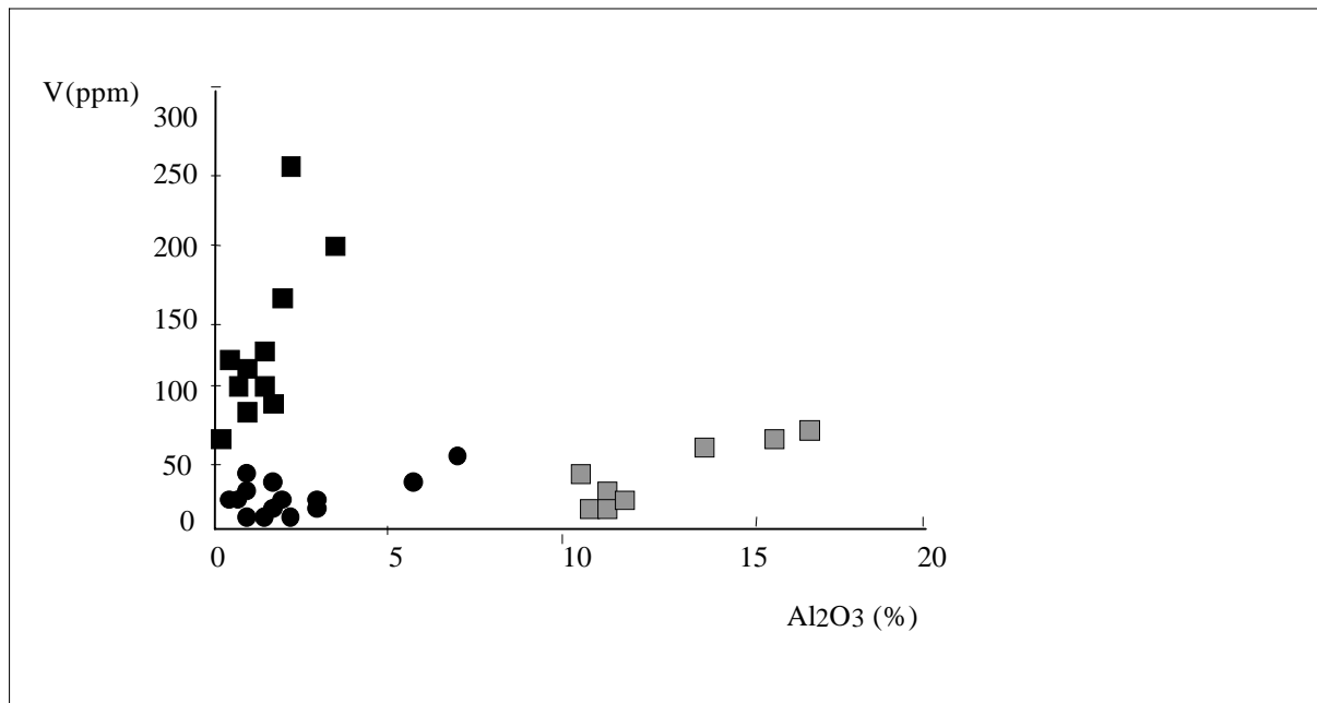
Abb. 27: A- Al 2 O 3 / Zr- und B- Al 2 O 3 / V-Verhältnis in Shales und Shaly BIF.
